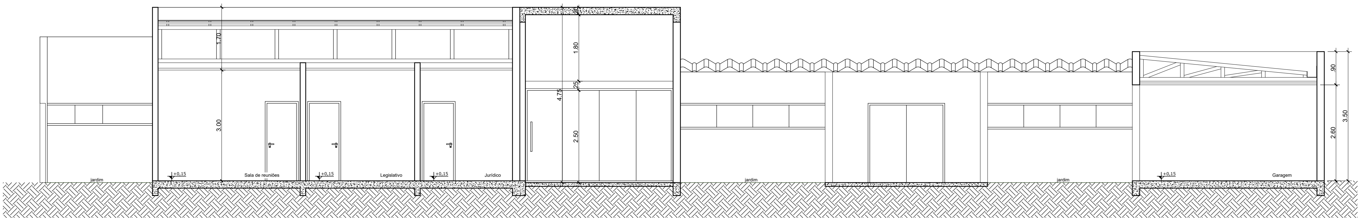
1 Corte AA *esboço para referência de alturas
